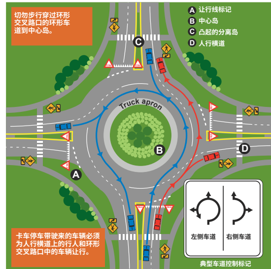
双车道环形交叉路口 (未反映所有的环形交叉路口设计)
